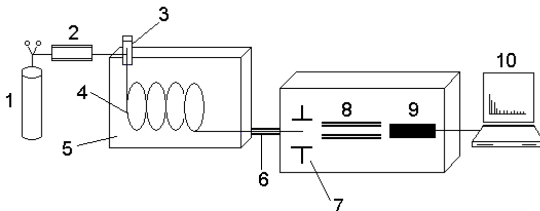
Rys. 65. Zestaw GC-MS: 1 - zbiornik gazu nośnego, 2 - regulator przepływu gazu, 3 - dozownik, 4 - kolumna, 5 - piec chromatograficzny, 6 - linia transferowa, 7 - źródło jonów, 8 - analizator (kwadropol), 9 - detektor, 10 - rejestrator (komputer)
