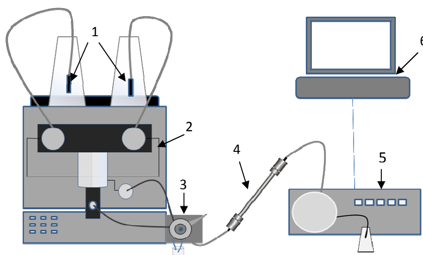
Rys. 68. Schemat chromatografu cieczowego, 1 – zbiornik fazy ruchomej, 2 – pompa, 3 – dozownik, 4 – kolumna chromatograficzna, 5 – detektor, 6 – komputer
