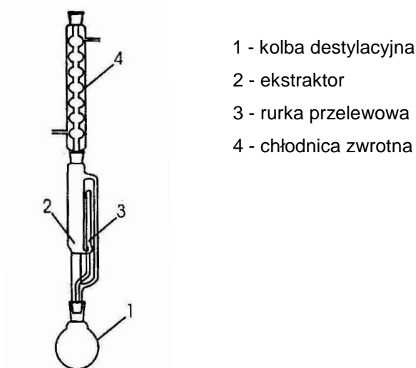
Rys. 46. Aparat Soxhleeta
