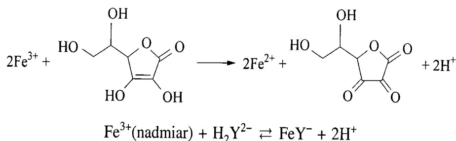
Rys. 80. Reakcja redukcji żelaza(III) do żelaza(II) kwasem askorbinowym
