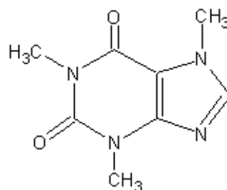
Rys. 99. Budowa chemiczna kofeiny
