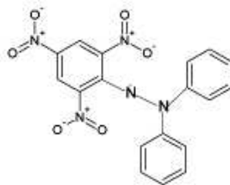
Rys. 85. Wzór DPPH
