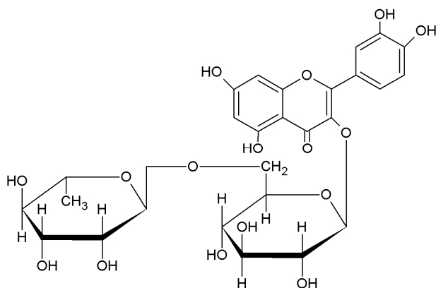
Rys. 42. Wzór rutyny
