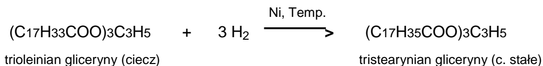
Rys. 12. Reakcja uwodornienia cząsteczki trioleinianu gliceryny
