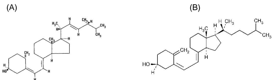
Rys. 15. Wzory witamin D: (A) ergokalcyferol, (B) cholekalcyferol
