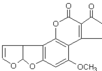
Rys. 31. Wzór aflatoksyne B 1
