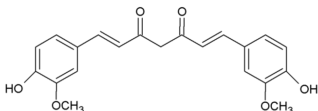
Rys. 41. Wzór kurkuminy
