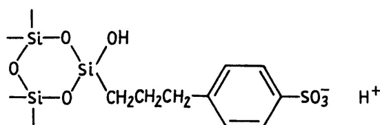
Rys. 72. Wymieniacz kationowy
