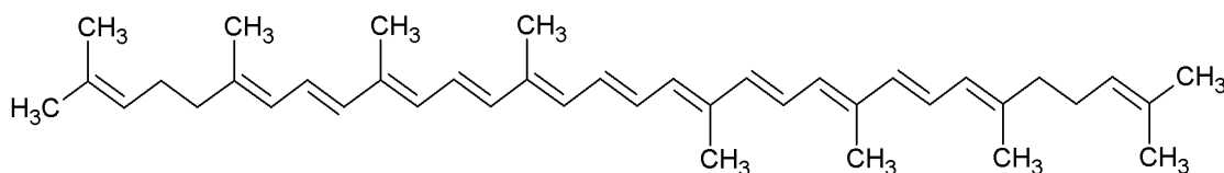
Rys. 40. Wzór likopenu
