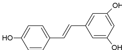
Rys. 39. Wzór resweratrolu
