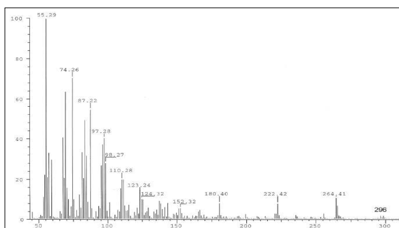
Widmo mas EI estru metylowego kwasu 1-oktadekenowego (18:1)
