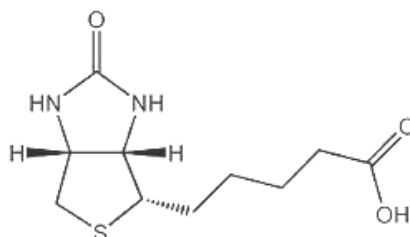
Rys. 26. Wzór biotyny
