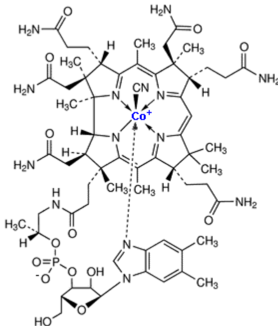
Rys. 25. Wzór cyjanokobalaminy
