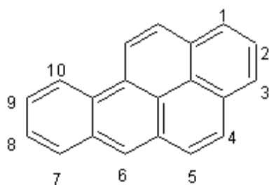
Rys. 32. Wzór benzo[a]pirenu
