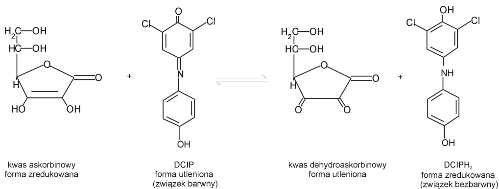
Rys. 78. Przebieg reakcji redukcji 2,6-dichlorofenoloindofenolu przez kwas L-askorbinowy
