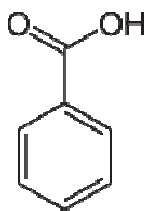
Rys. 100. Budowa chemiczna kwasu benzoowego
