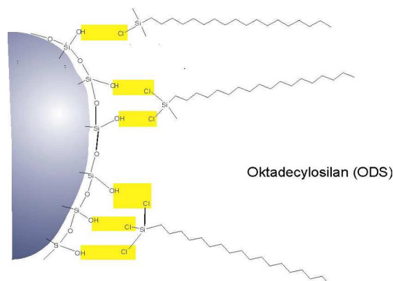
Rys. 70. Faza oktadecylosilanowa
