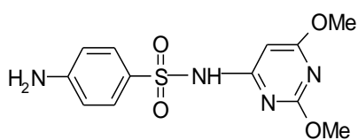
Rysunek 2. Budowa chemiczna i wybrane parametry fizykochemiczne sulfadimetoksyny
